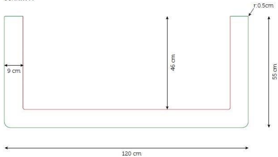
Schnitt A
