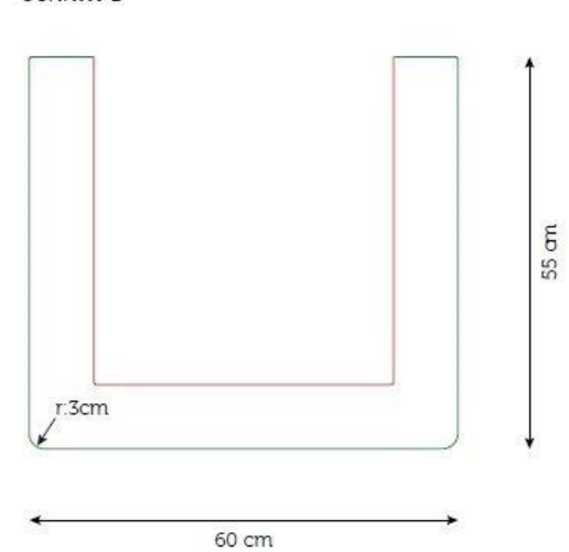
Schnitt B
