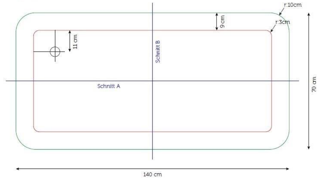
Grundriss
